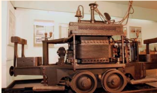
Die erste elektrische Grubenlok der Welt, genannt Dorothea.
